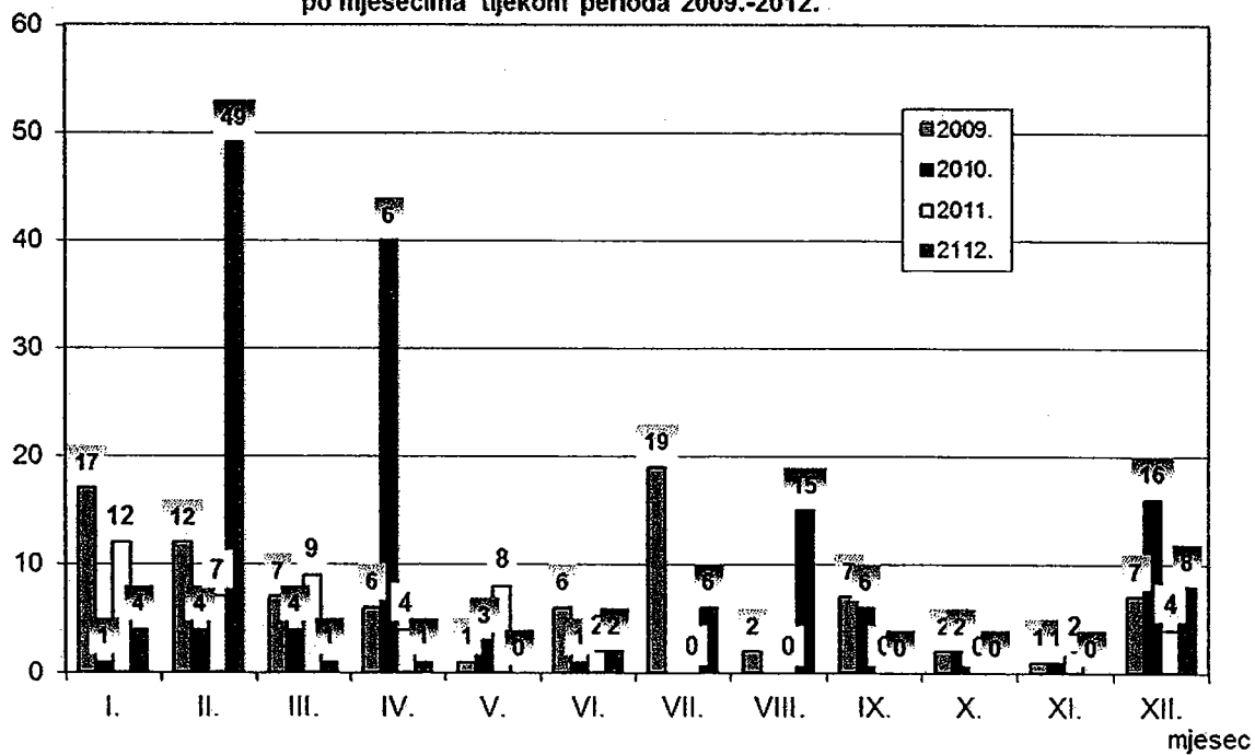
Sisak-1: usporedba broja prekoračenja satnih koncentracija H_2S > GV po mjesecima tijekom perioda 2009.-2012.
