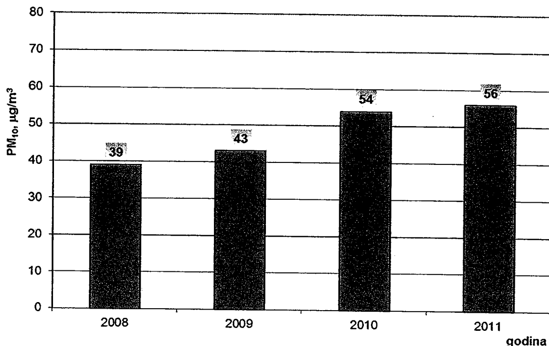
Sisak-1: srednje godišnje koncentracije PM 10 tijekom perioda 2008.-2011. PM 10 > 52 mg/m 3 (2008.), 48 mg/m 3 (2009.), 44 mg/m 3 (2010.), 40 mg/m 3 (2011.), gravimetrijska metoda
