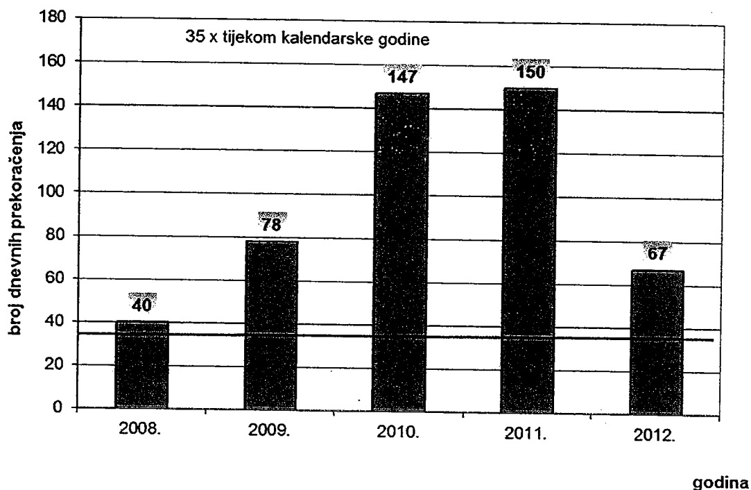
Sisak-1: broj prekoračenja dnevnih koncentracija PM 10 > 50 mg/m 3 , gravimetrijska metoda u periodu 2008.-2012.
