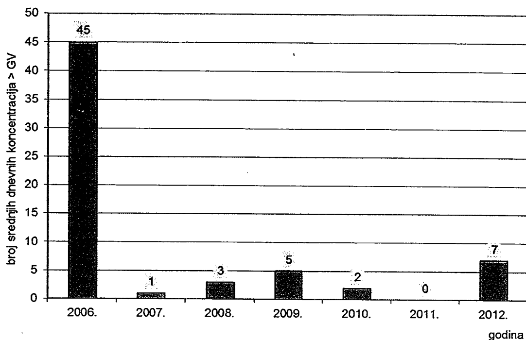
Sisak-1: broj prekoračenja srednjih dnevnih koncentracija \text{H}_2\text{S} > 5 \mu\text{g}/\text{m}^3 u periodu 2006.-2012.
