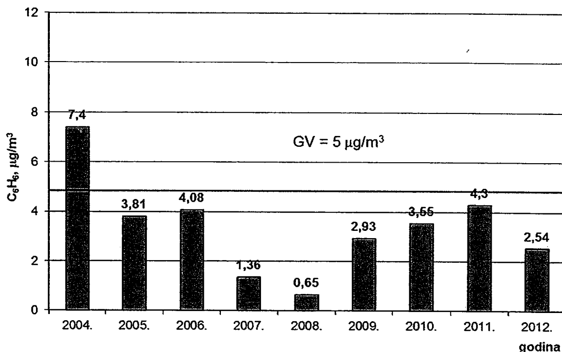
Sisak-1: srednje godišnje koncentracije C 6 H 6 u periodu 2004.-2012.
