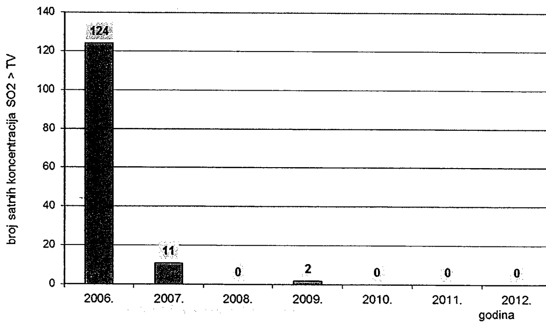
Sisak-1 : broj prekoračenja satnih koncentracija \text{SO}_2 > 500 (2006.), 470 (2007.), 440 (2008.), 410 (2009.), 380 (2010.), 350 (2011. i 2012.) / \mu\text{g}/\text{m}^3
